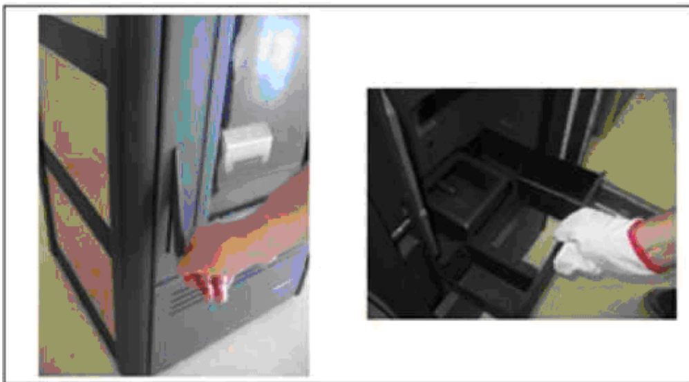
Фигура 6.5. Почистване на пепелника.
