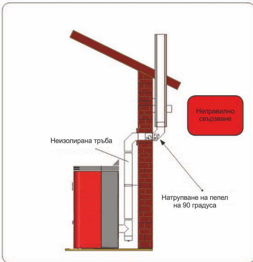
Фигура 3.5. Вътрешен/външен монтаж на комина – неправилно свързване.
